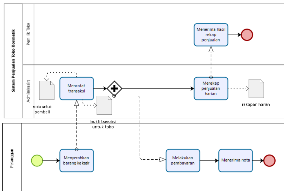
Gambar 3. 1 BPMN Prosedur yang Sedang Berjalan
