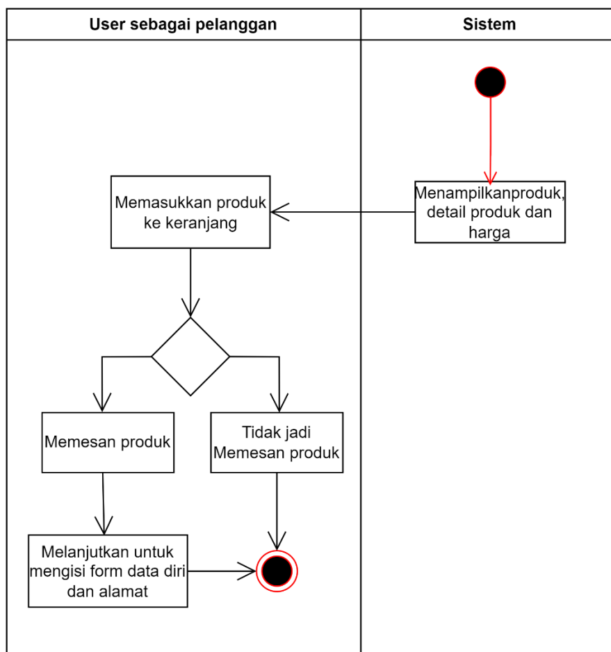
Gambar 3. 15 Activity Diagram proses memilih produk
