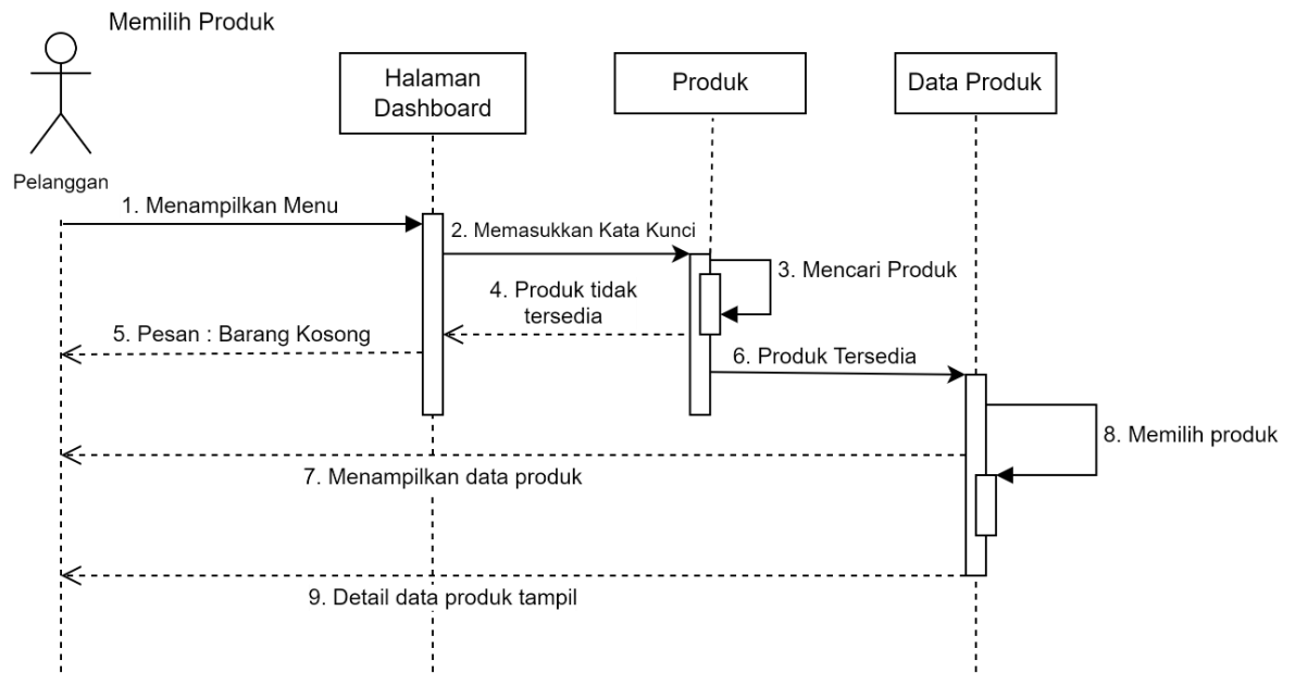
Gambar 3. 7 Sequence Diagram Memilih Produk
