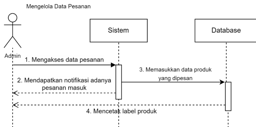
Gambar 3. 10 Sequence Diagram Mengelola Data Pesanan
