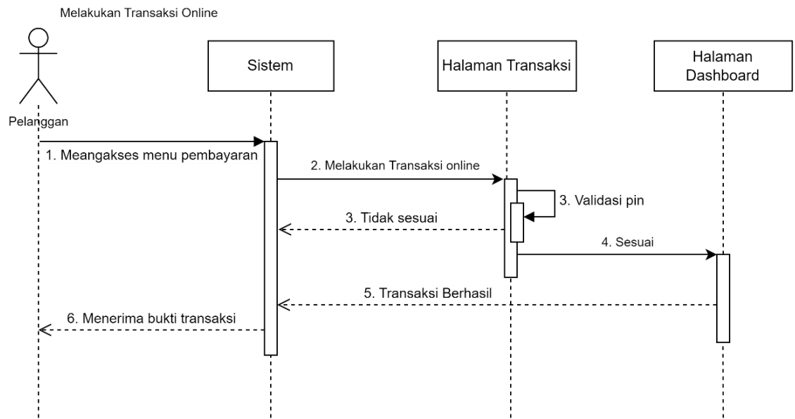
Gambar 3. 9 Sequence Diagram Melakukan Transaksi Online
