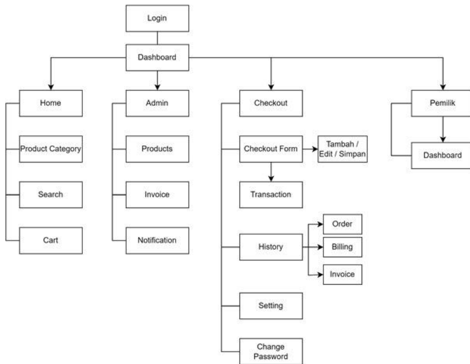
Gambar 3. 22 Struktur Menu
