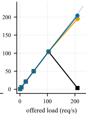
MobileNetV2
