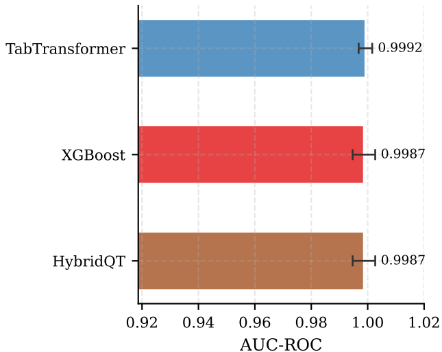
CKD Dataset
