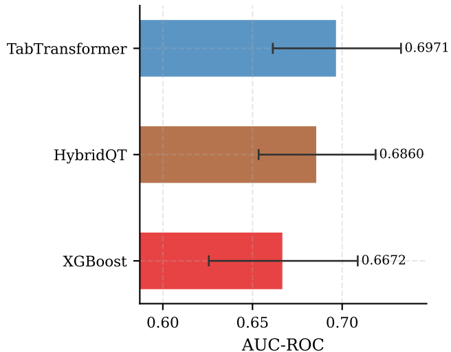
FHS Dataset
