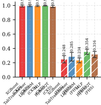
F1 Score
