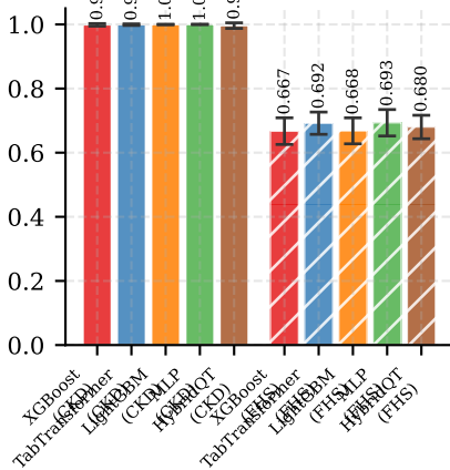
AUC-ROC
