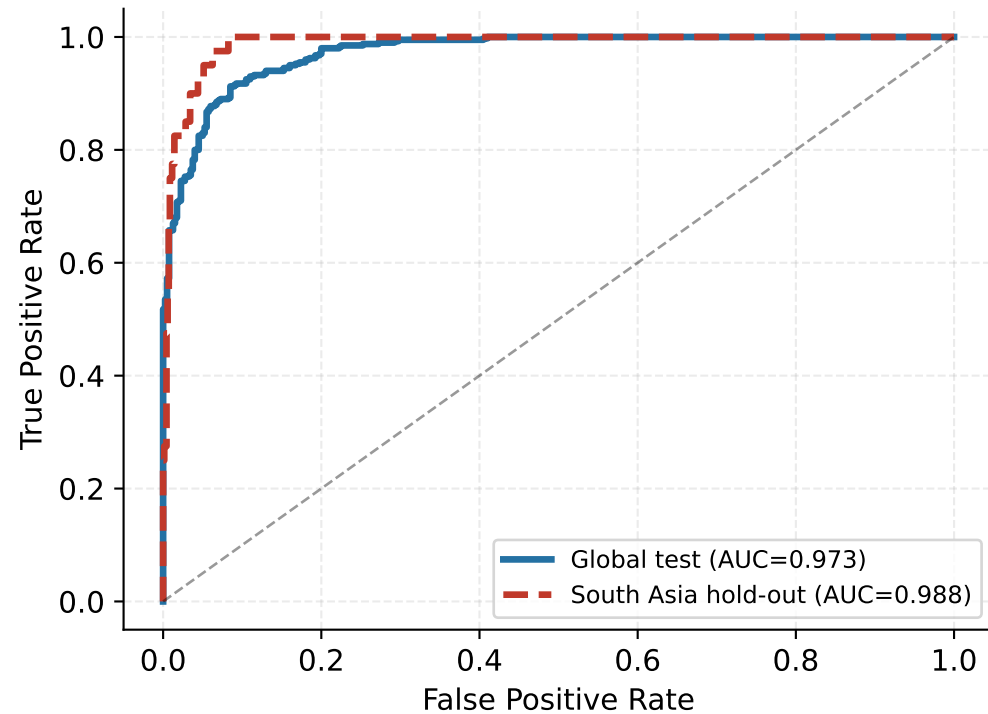
A ROC Curves: Global vs SA Hold-Out
