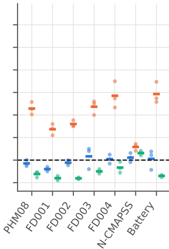
nominal \alpha = 0.10
