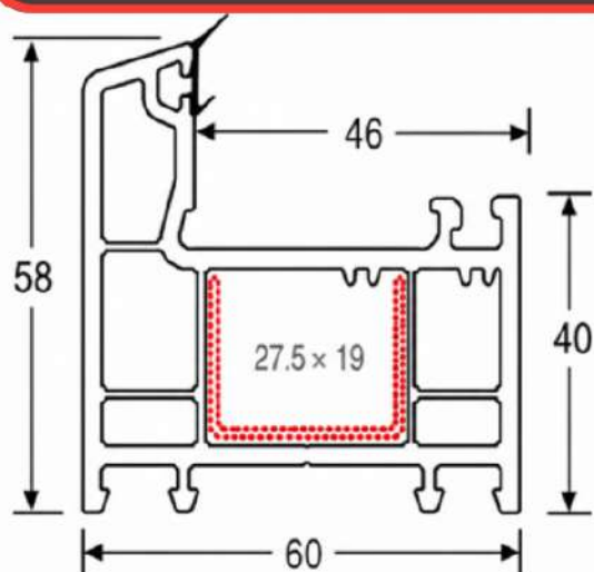
60 Frame D2
