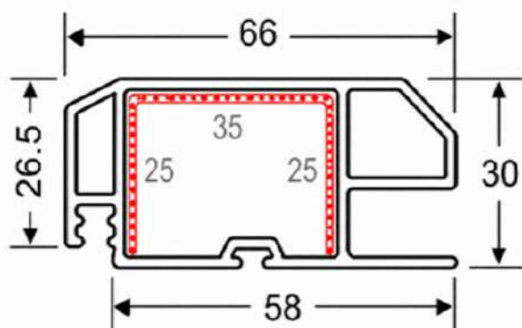
66 Screen Door Sash
