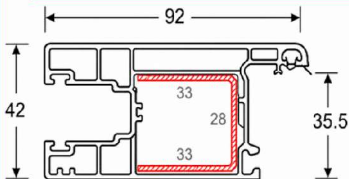
60 Sliding Door Sash A8
