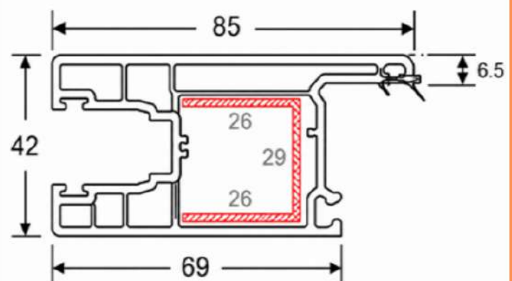
60 Sliding Door Sash 3
