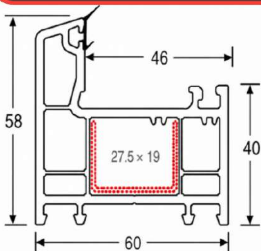
60 Frame D2
