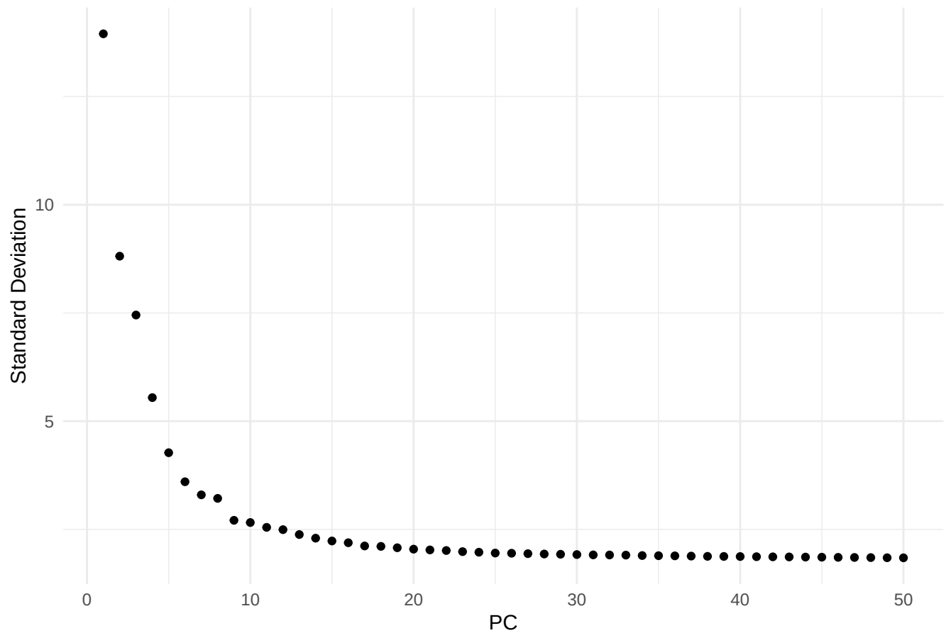
Elbow plot – choix des composantes principales
