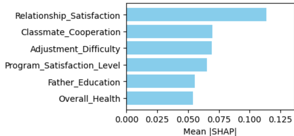
CatBoost
