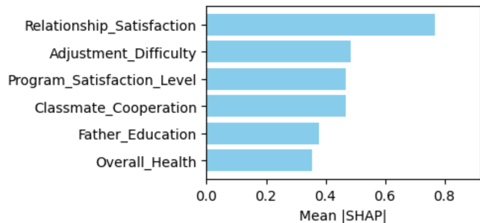
CatBoost
