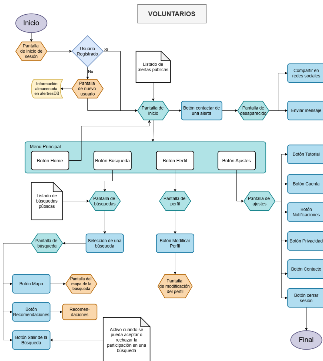
Figura 4.4: Diagrama navegacional del prototipo creado para el perfil de voluntarios. Fuente propia.
