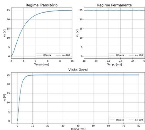
Figura 41 – Tensão no capacitor do conversor Buck alternativo.
