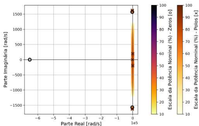
Figura 43 – Posição dos polos e zeros do sistema de controle do projeto alternativo para diferentes níveis de potência de operação.
