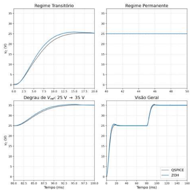
Figura 49 – Comparação do Sinal v_C do conversor Buck alternativo: Simulação Numérica ( n = 100 ) vs. QSPICE.
