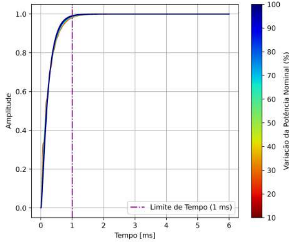
Figura 21 – Resposta transitória do sistema em função da variação da potência nominal
