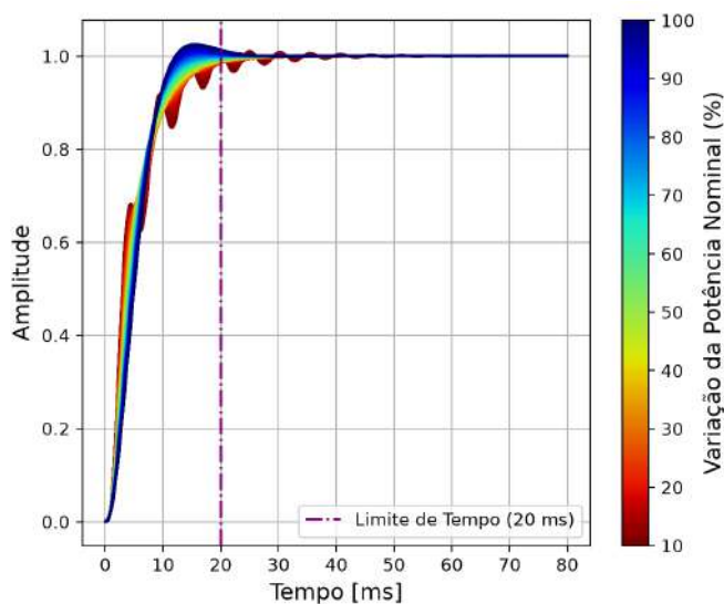
Figura 44 – Resposta transitória do sistema de controle do projeto alternativo para diferentes níveis de potência de operação.
