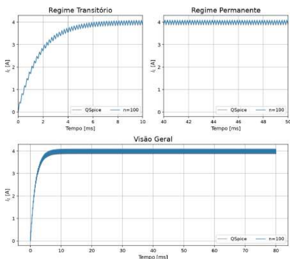
Figura 40 – Corrente no indutor do conversor Buck alternativo.
