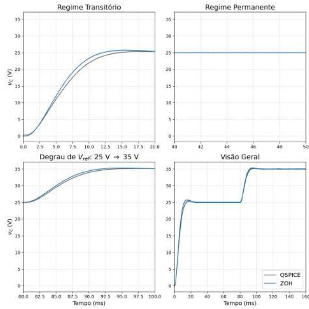
Figura 47 – Comparação do Sinal v_C do conversor Buck alternativo: Simulação Numérica ( n = 1000 ) vs. QSPICE.
