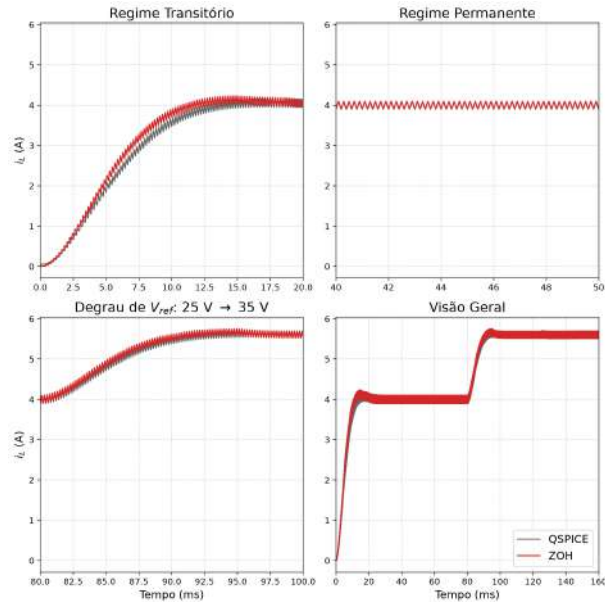
Figura 48 – Comparação do Sinal i_L do conversor Buck alternativo: Simulação Numérica ( n = 100 ) vs. QSPICE.
