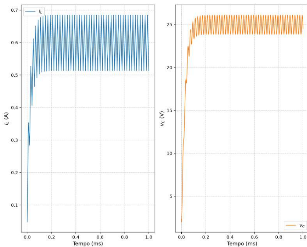
Figura 39 – Simulação QSPICE da corrente no indutor e tensão no condensador do conversor Buck projetado.
