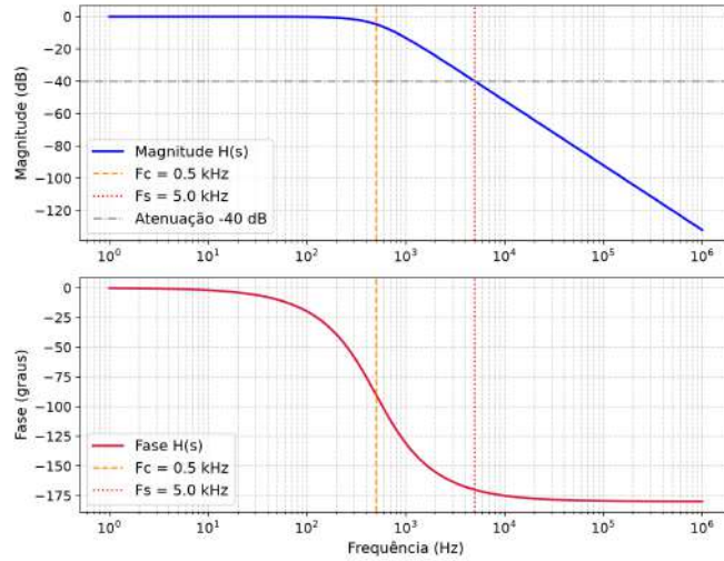
Figura 42 – Diagrama de Bode da resposta em frequência do filtro antialiasing do conversor Buck alternativo.
