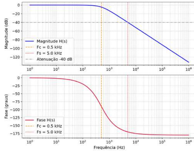
Figura 39 – Diagrama de Bode da resposta em frequência do filtro antialiasing do conversor Buck alternativo.
