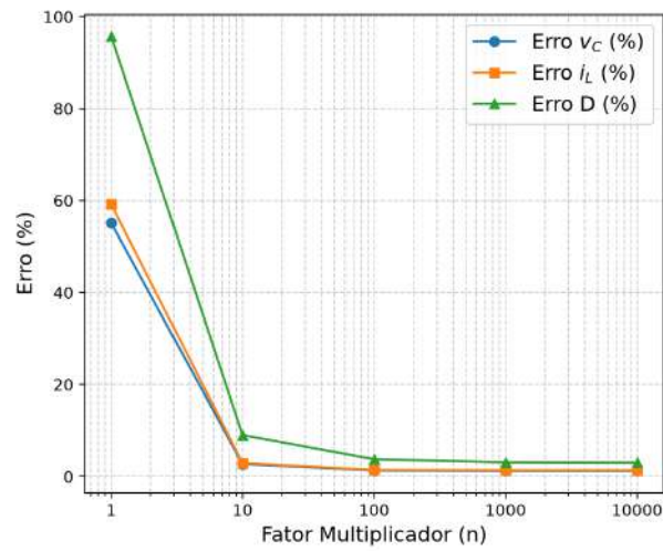
Figura 42 – Erro relativo percentual médio em malha fechada alternativo da corrente ( i_L ), da tensão ( v_C ) e duty cycle ( D ) em função do fator n , tendo o QSPICE como referência.
