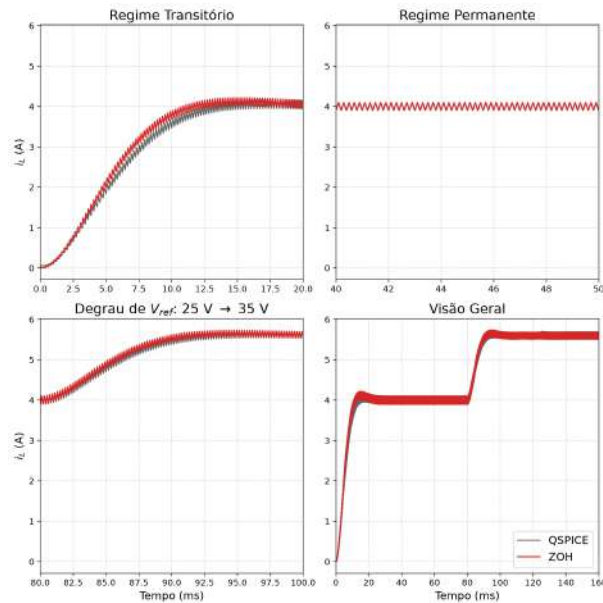
Figura 43 – Comparação do Sinal i_L do conversor Buck alternativo: Simulação Numérica ( n = 1000 ) vs. QSPICE.
