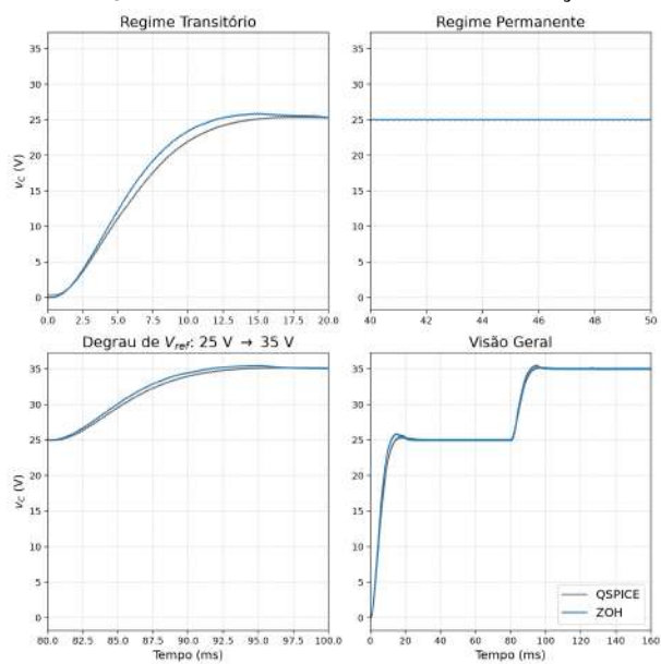
Figura 46 – Comparação do Sinal v_C do conversor Buck alternativo: Simulação Numérica ( n = 100 ) vs. QSPICE.
