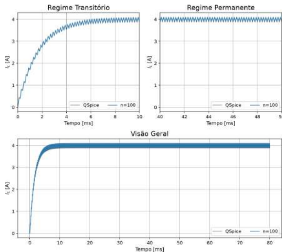
Figura 37 – Corrente no indutor do conversor Buck alternativo.
