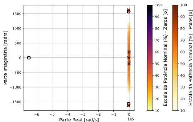
Figura 40 – Posição dos polos e zeros do sistema de controle do projeto alternativo para diferentes níveis de potência de operação.
