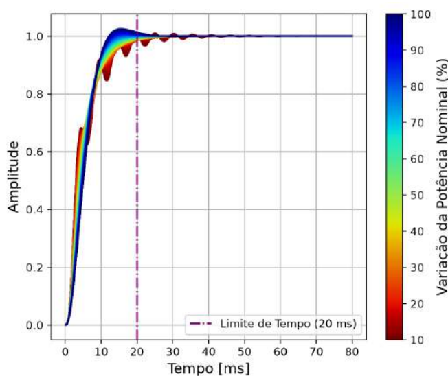
Figura 41 – Resposta transitória do sistema de controle do projeto alternativo para diferentes níveis de potência de operação.
