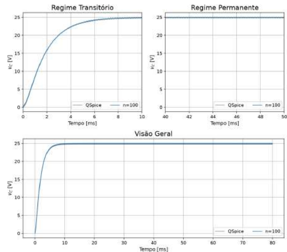
Figura 38 – Tensão no capacitor do conversor Buck alternativo.
