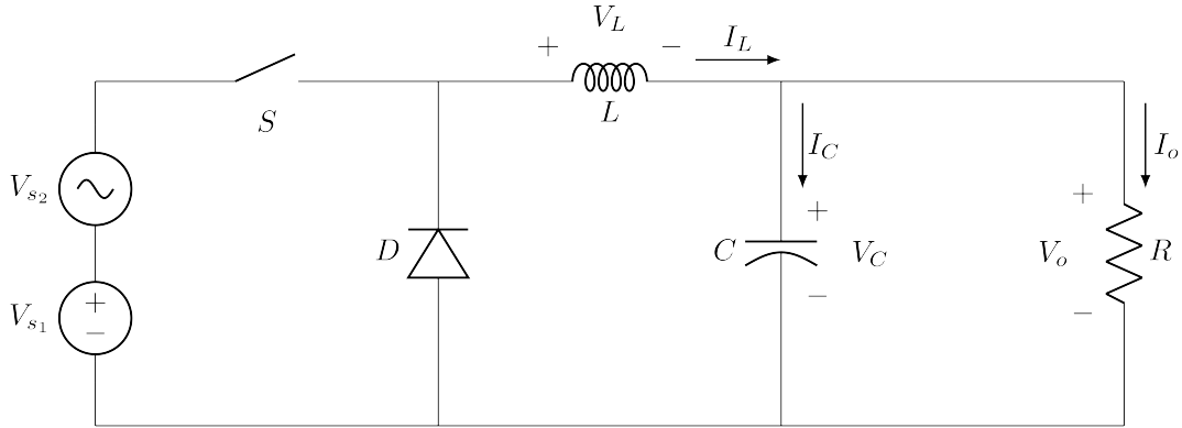
Figura 4 – Topologia do circuito conversor Buck
