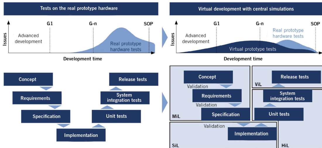
Figura 1 – Comparação entre o Ciclo em V tradicional e sua evolução baseada em MBD
