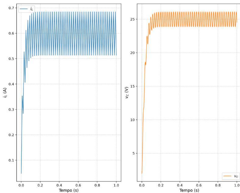
Figura 36 – Simulação QSPICE da corrente no indutor e tensão no condensador do conversor Buck projetado.
