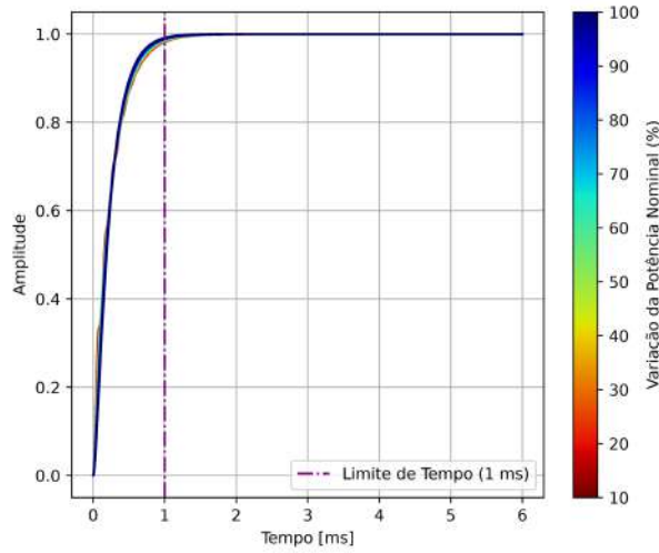
Figura 21 – Resposta transitória do sistema em função da variação da potência nominal
