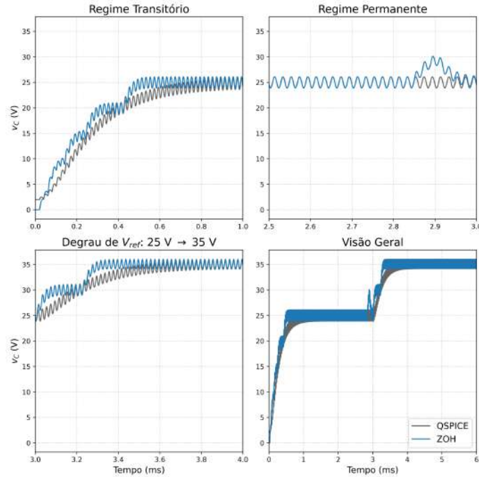
Figura 23 – Comparação do Sinal v_C : Simulação Numérica ( n = 10 ) vs. QSPICE
