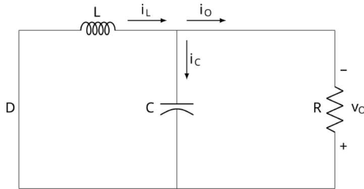
Figura 7 – Circuito equivalente com a chave aberta
