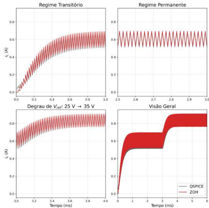
Figura 29 – Comparação do Sinal i_L : Simulação Numérica ( n = 1000 ) vs. QSPICE
