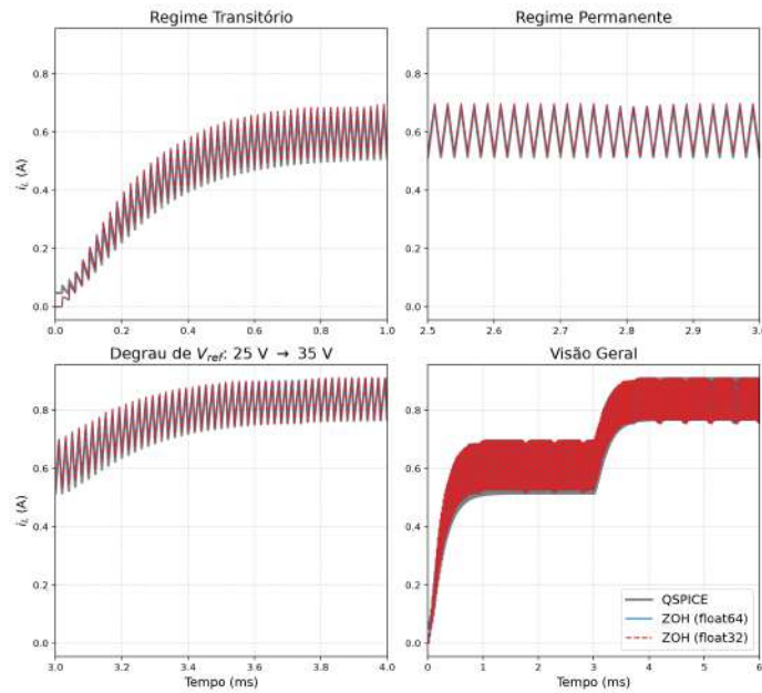
Figura 30 – Comparação do sinal de corrente no indutor i_L : Precisão Simples ( float32 ) vs. Dupla ( float64 ) e Referência QSPICE
