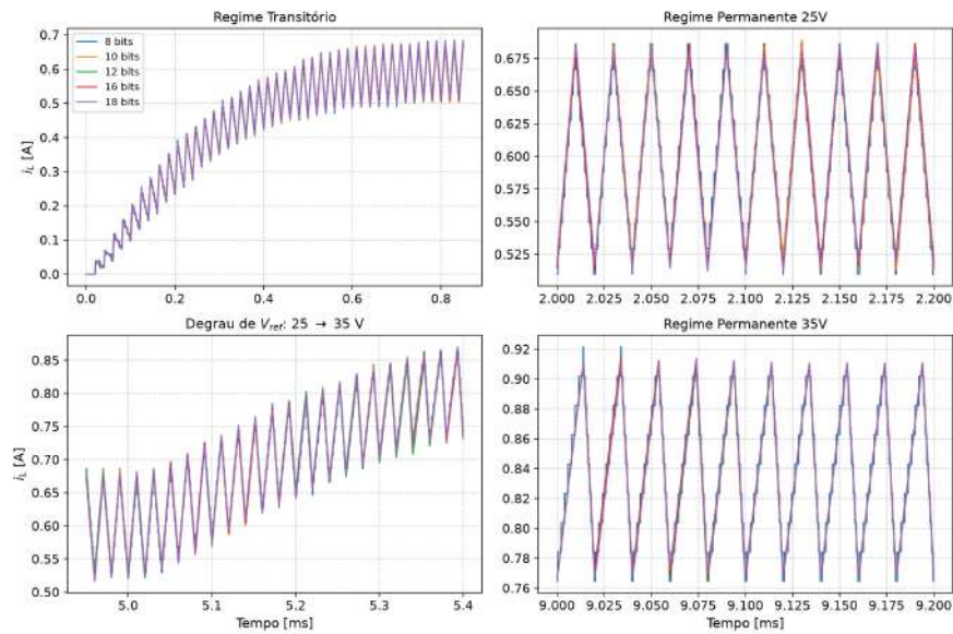
Figura 34 – Detalhamento da corrente no indutor ( i_L ) em diferentes etapas de operação em função da resolução do DAC.
