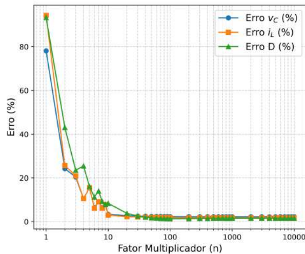
Figura 25 – Erro relativo percentual médio em malha fechada da corrente ( i_L ), da tensão ( v_C ) e duty cycle ( D ) em função do fator n , tendo o QSPICE como referência
