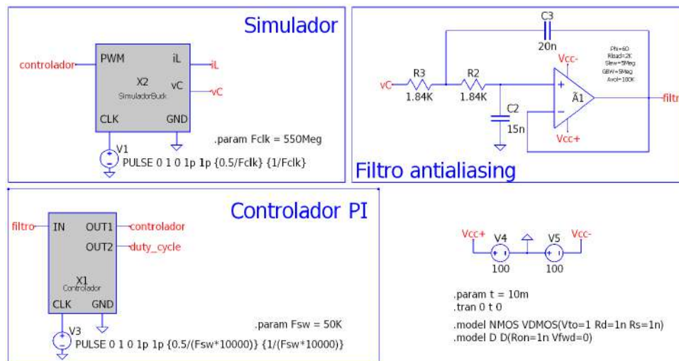
Figura 32 – Circuito com simulação do simulador do Buck implementado em microcontrolador no QSPICE.
