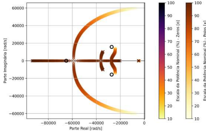
Figura 20 – Posição dos polos e zeros do sistema em função da variação da potência nominal
