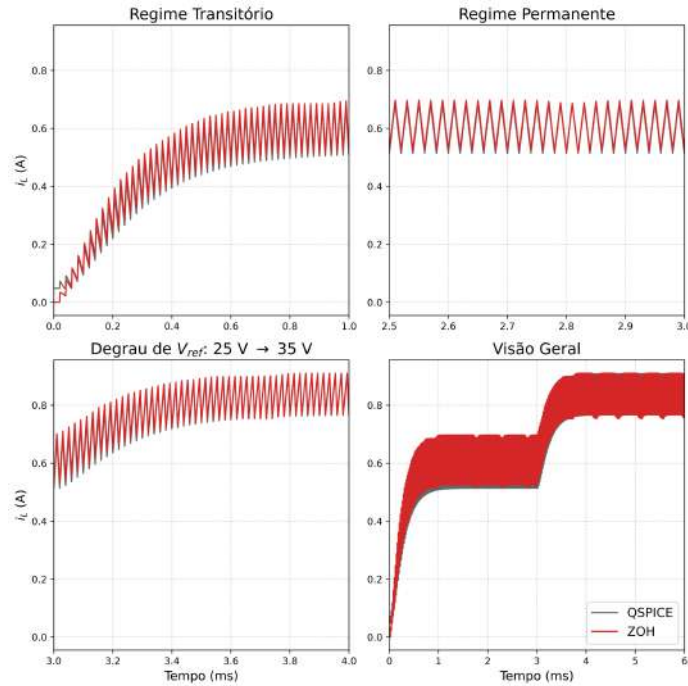
Figura 27 – Comparação do Sinal i_L : Simulação Numérica ( n = 100 ) vs. QSPICE
