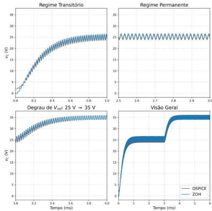
Figura 28 – Comparação do Sinal v_C : Simulação Numérica ( n = 1000 ) vs. QSPICE
