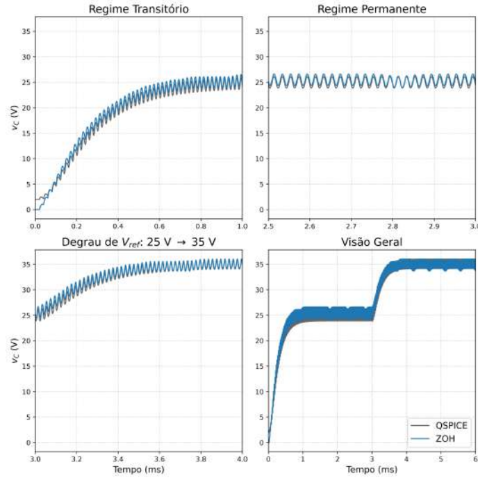
Figura 26 – Comparação do Sinal v_C : Simulação Numérica ( n = 100 ) vs. QSPICE
