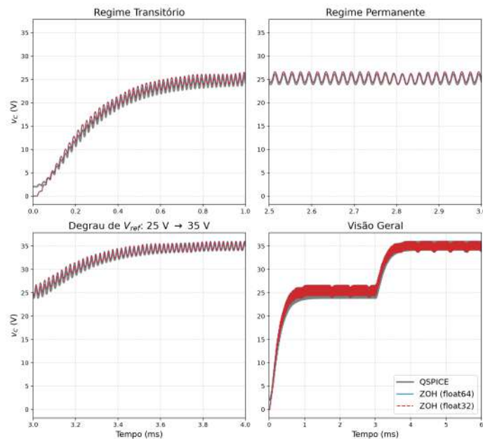
Figura 31 – Comparação do sinal de tensão no capacitor v_C : Precisão Simples ( float32 ) vs. Dupla ( float64 ) e Referência QSPICE
