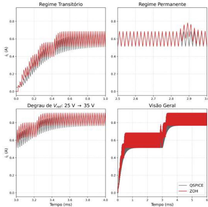
Figura 24 – Comparação do Sinal i_L : Simulação Numérica ( n = 10 ) vs. QSPICE
