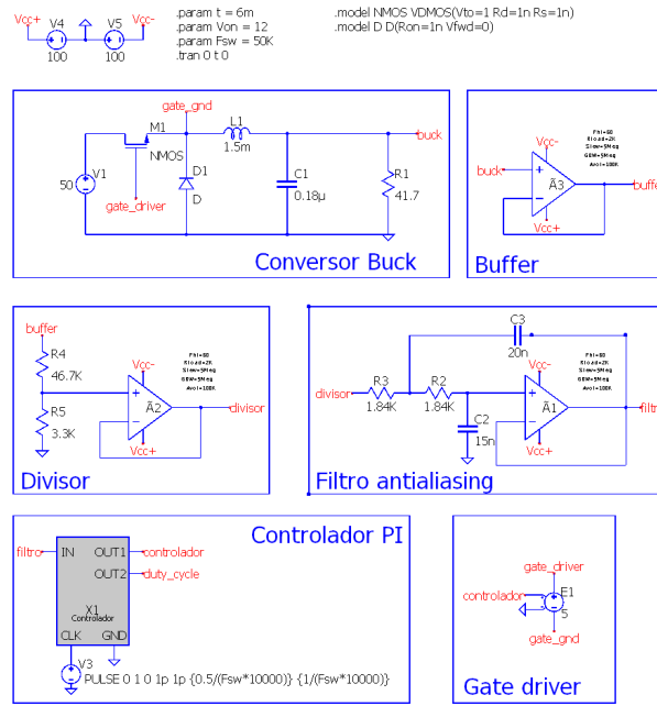
Figura 22 – Circuito do conversor Buck em malha fechada implementado no QSPICE
