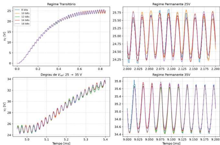
Figura 35 – Detalhamento da tensão no capacitor ( v_C ) em diferentes etapas de operação em função da resolução do DAC.
