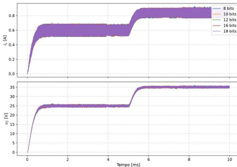
Figura 33 – Comportamento completo da corrente no indutor e tensão no capacitor para diferentes resoluções do DAC.
