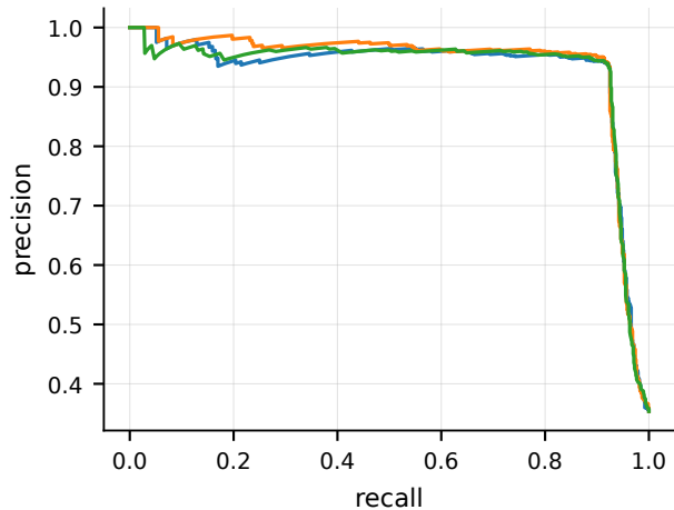
Precision--Recall
