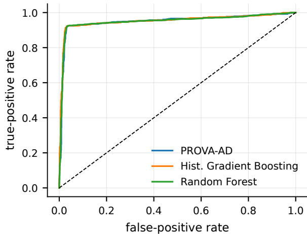
ROC
