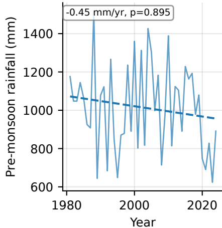
CHIRPS Sylhet 1981-2024
