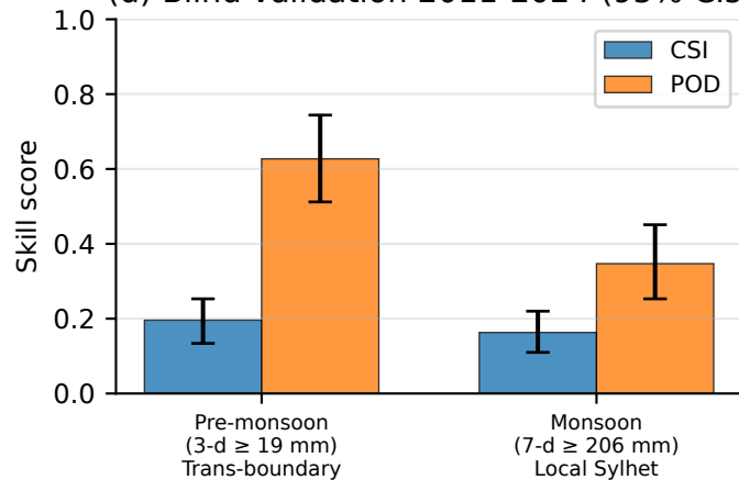
(d) Blind validation 2011-2024 (95% CIs)
