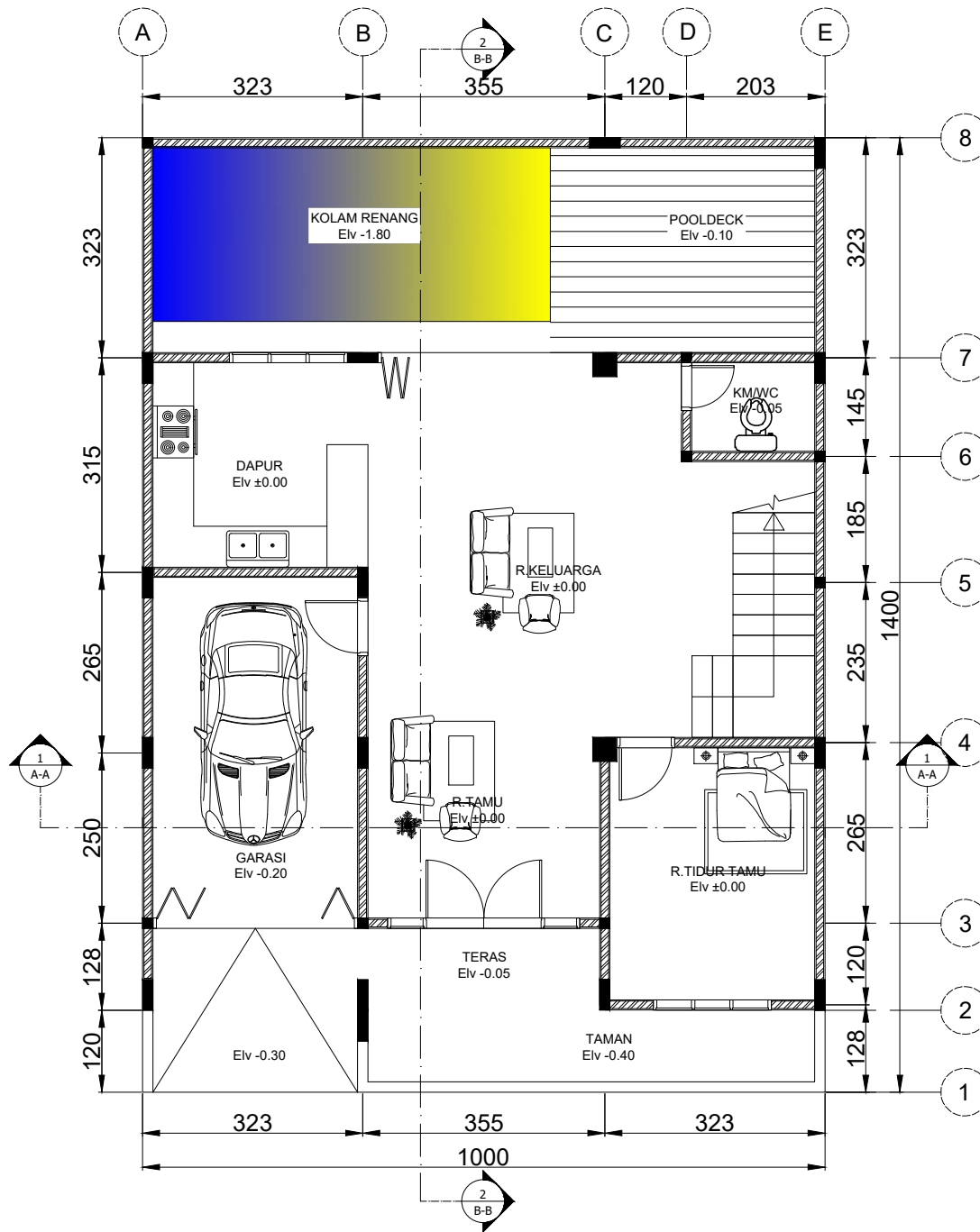
1 DENAH LANTAI 1 Scale: 1:100
