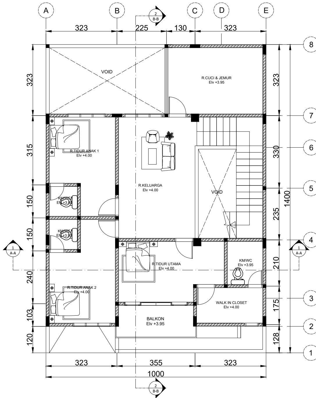
2 DENAH LANTAI 2 Scale: 1:100
