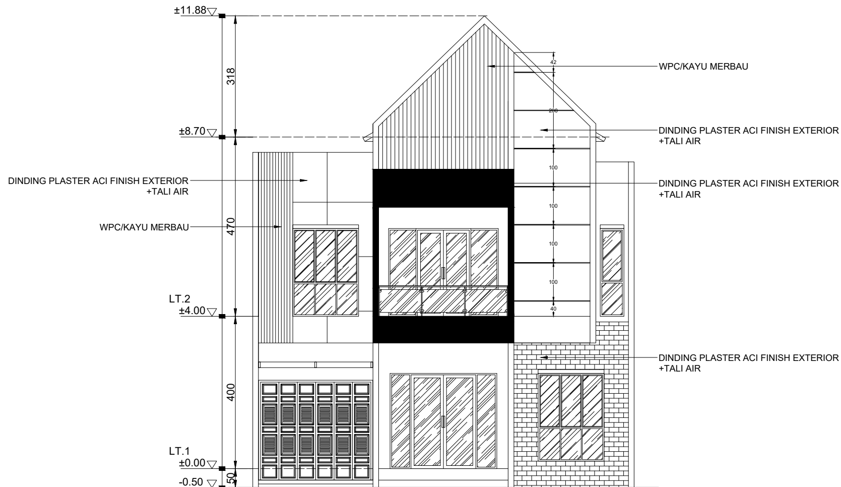
5 TAMPAK DEPAN Scale: 1:100
