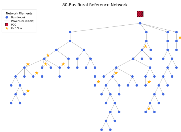
รูปที่ 3. Grid bus network topology used for simulator.
