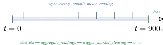
รูปที่ 7. ลำดับเวลาการเคลียร์ตลาดของโปรแกรม oracle: ค่าอ่านที่ลงนามแล้วทยอยเข้ามาตลอดหน้าต่างรวมข้อมูล 15 นาที (900 วินาที) เมื่อหน้าต่างปิด oracle จะรวมค่าอ่าน ส่งเคลียร์ตลาด แล้วชำระคู่ที่จับคู่ได้บนเชน ทั้งนี้เป็นเส้นทาง telemetry บนเชนตามที่ออกแบบและที่วัดแบบแยกส่วนในหัวข้อ X.H.4 ส่วนสายงานที่ติดตั้งใช้งานจริงไม่ได้เขียนค่าอ่านลงเชน แต่จับเส้นทาง ingest ไว้ที่ Redis Streams และส่งหน้าต่างเวลาในรูปที่ 4 แล้วจึงแกะเฉพาะตอน mint และตอนชำระธุรกรรมเท่านั้น
