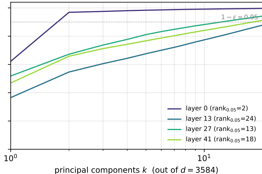
Gemma-2-9B-it
