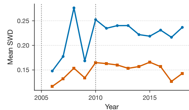
AE-latent SWD
