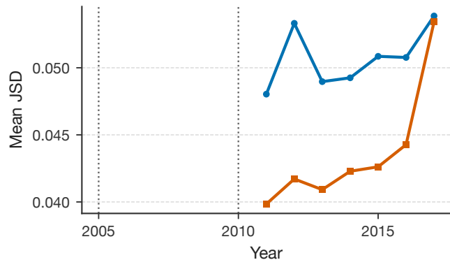
AE-latent SWD
