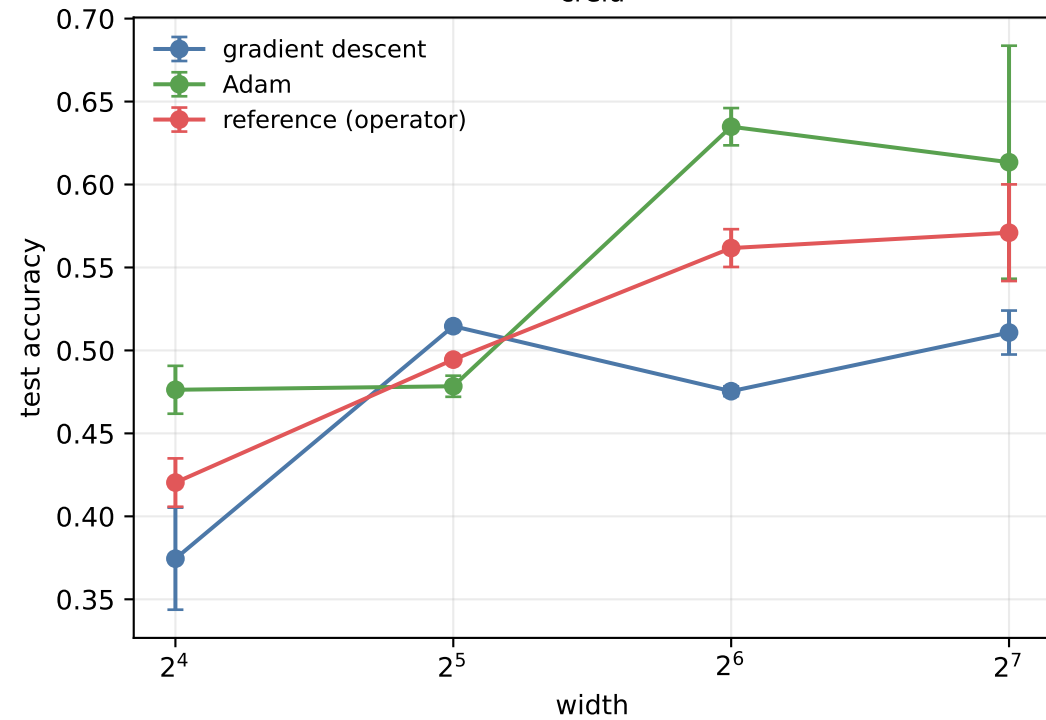
crelu
