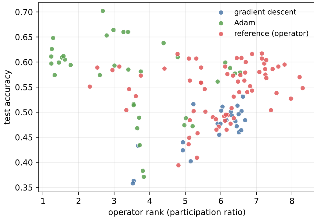
crelu
