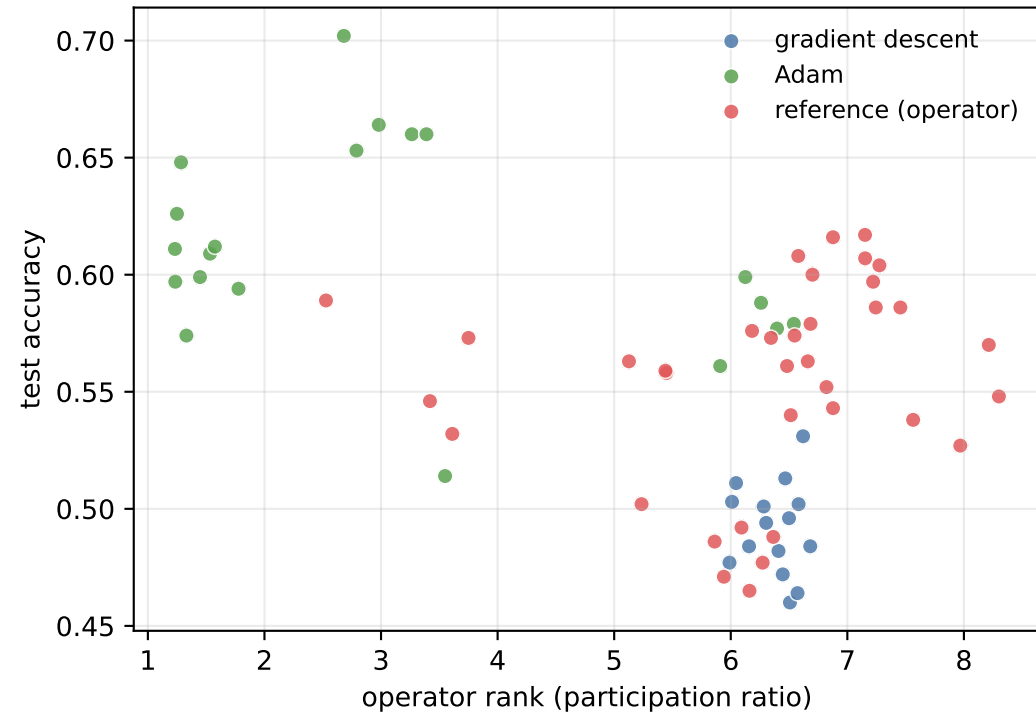
crelu
