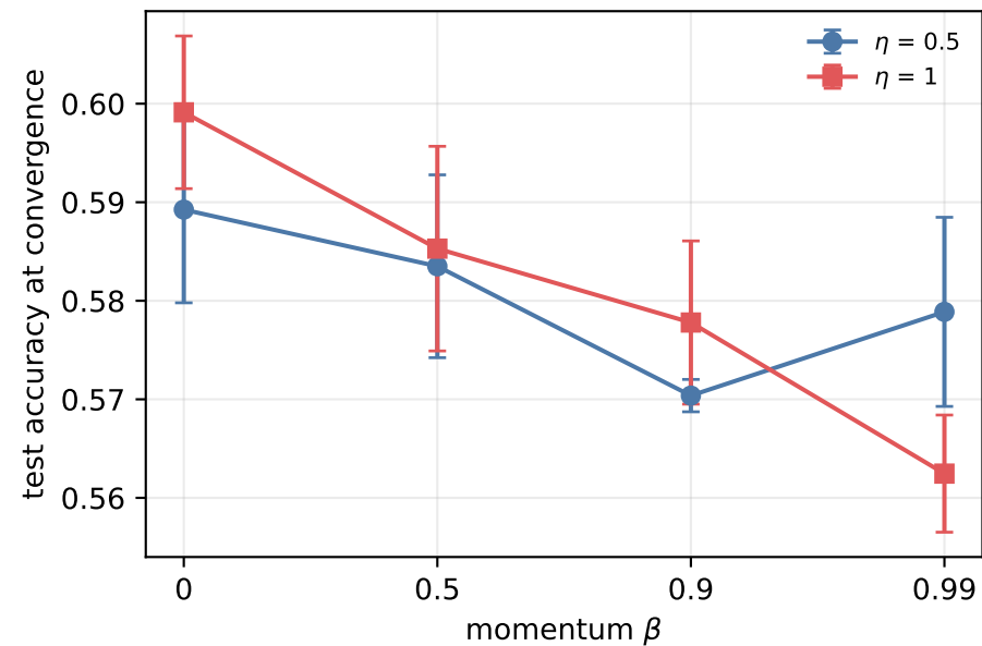
crelu: generalisation
