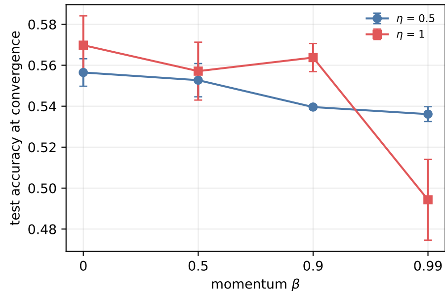
relu: generalisation
