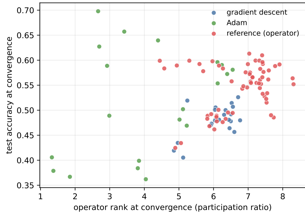
crelu
