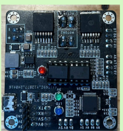
Hình 12: Mạch in PCB
