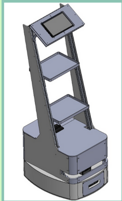
Hình 1: Tổng quan robot
