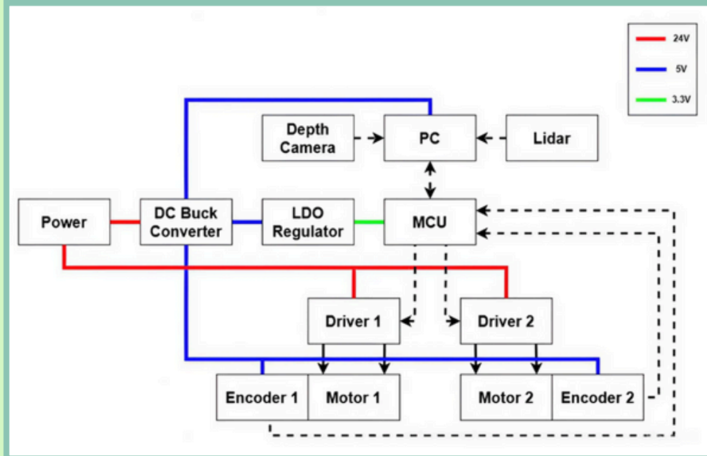
Hình 2: Tổng quan hệ thống điện
