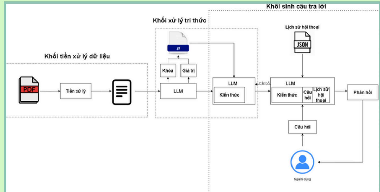
Hình 6: Kiến trúc hệ thống AI
