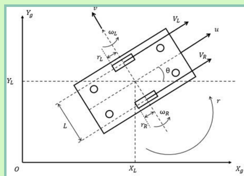
Hình 4: Mô hình động học trên bánh xe
