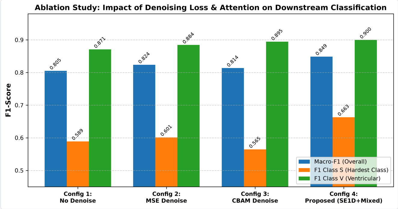
Hình 8: So sánh Hiệu năng Phân loại F1-Score giữa 4 Cấu hình Ablation Study Kiểm chứng Chéo.
