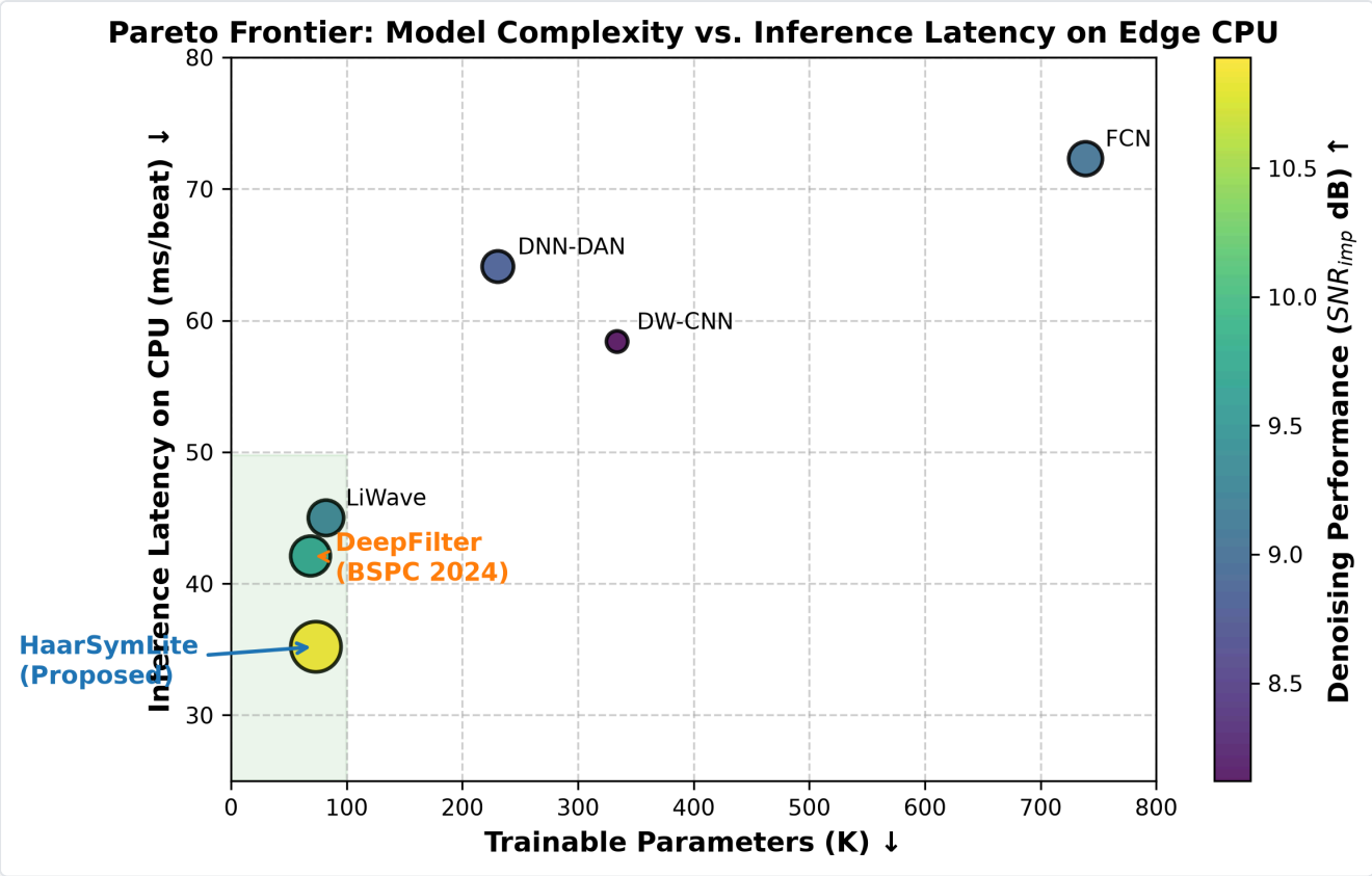
Hình 9: Đồ thị Biên Pareto: Đánh đổi giữa Độ phức tạp Mô hình (Tham số) và Độ trễ Suy luận trên CPU Tiêu chuẩn.
