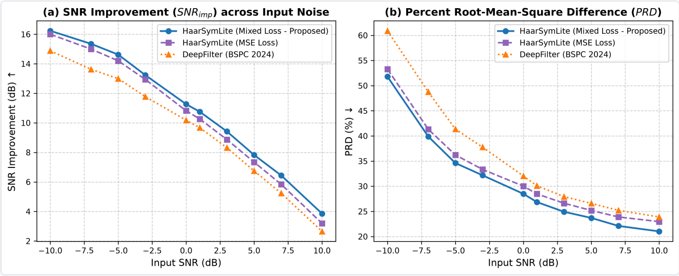
Hình 4: Đồ thị So sánh Mức Cải thiện SNR ( SNR_{imp} dB) và Độ Biến dạng PRD (%) trên Toàn dải Nhiễu (từ -10 dB đến +10 dB).
