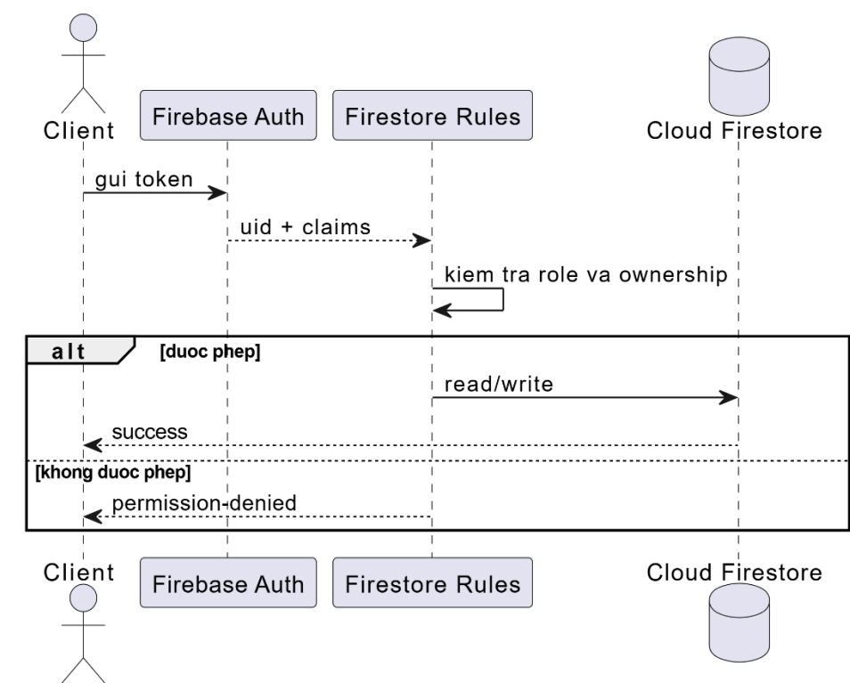
Hình 10. Sơ đồ luồng phân quyền và bảo mật dữ liệu
