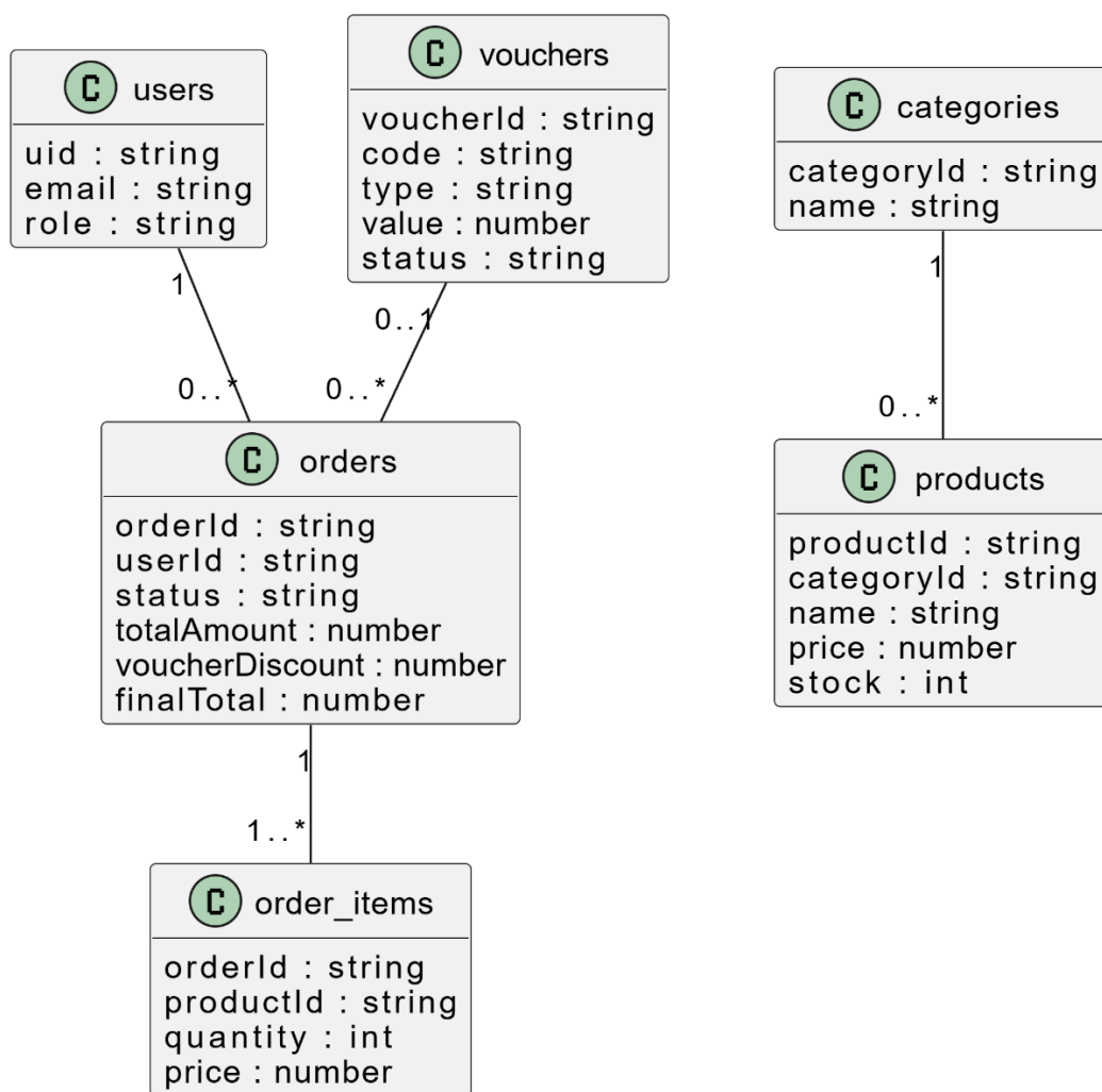
Hình 3. Sơ đồ dữ liệu logic (ERD)
