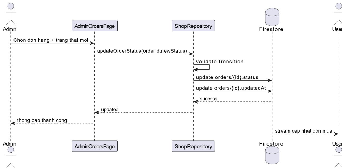
Hình 6. Sơ đồ tuần tự admin cập nhật trạng thái đơn hàng
