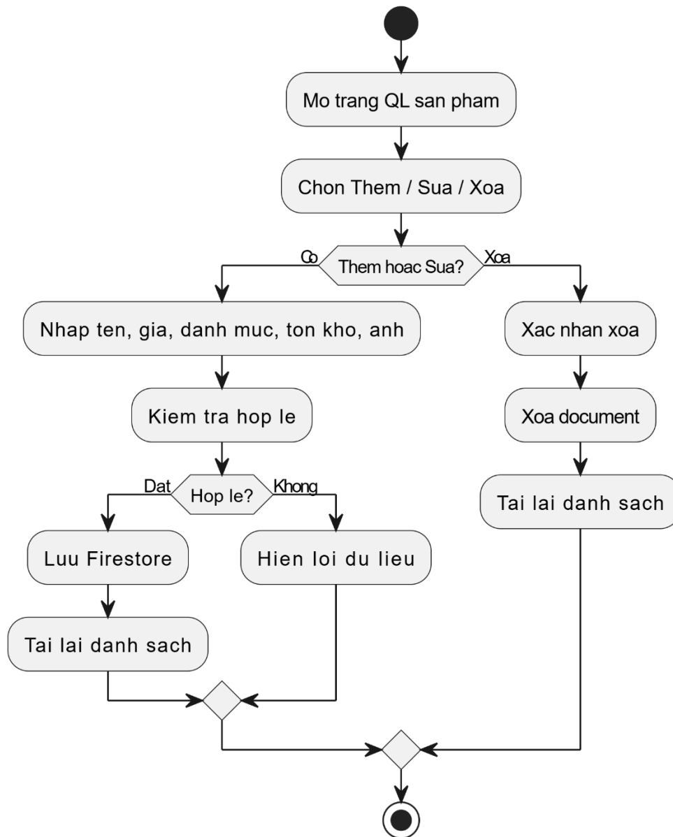
Hình 8. Sơ đồ hoạt động CRUD sản phẩm (Admin)
