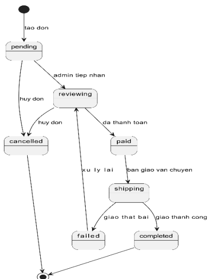
Hình 7. Sơ đồ trạng thái đơn hàng (State Machine)
