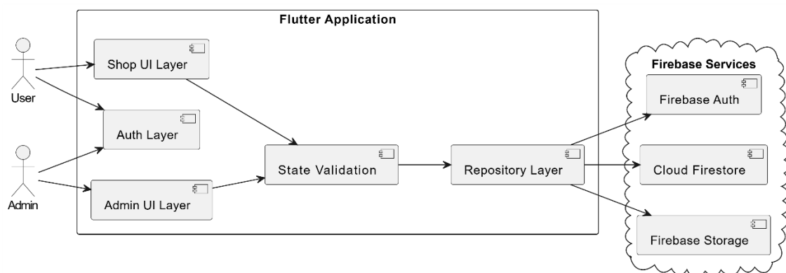
Hình 2. Kiến trúc tổng thể
