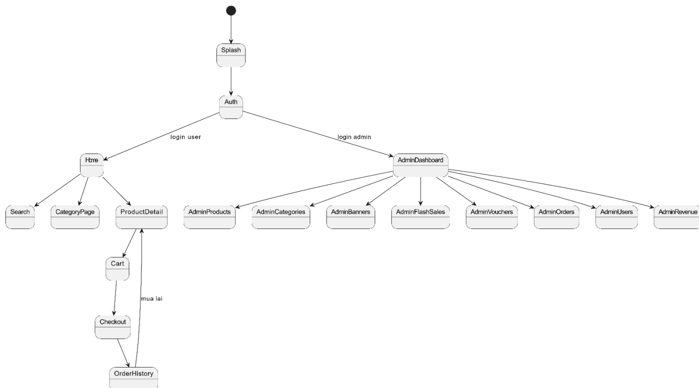
Hình 9. Sơ đồ điều hướng màn hình (Navigation Flow)
