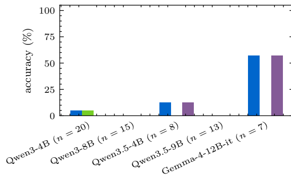
(b) AIME 24&amp;25
