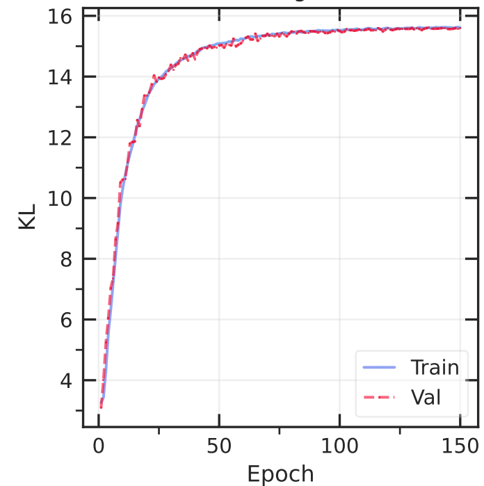
KL Divergence
