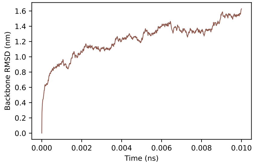
PfATP4-WT (ligand 438)
