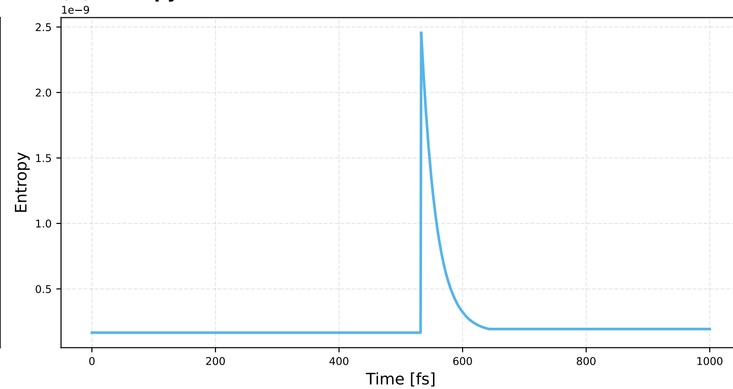
(d) Entropy Evolution
