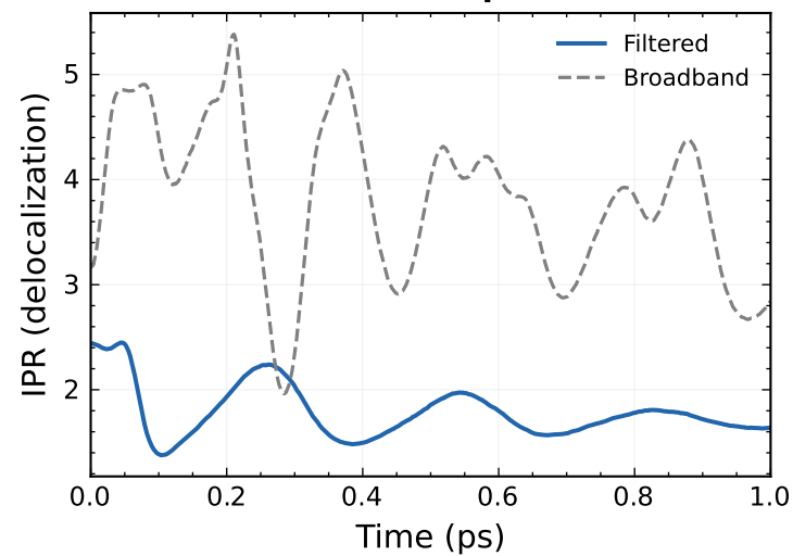
(d) Inverse Participation Ratio
