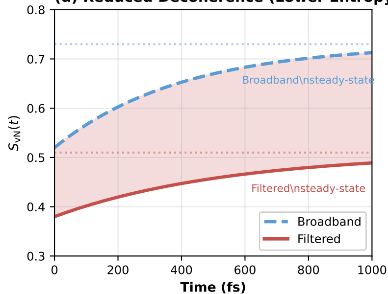
(d) Reduced Decoherence (Lower Entropy)
