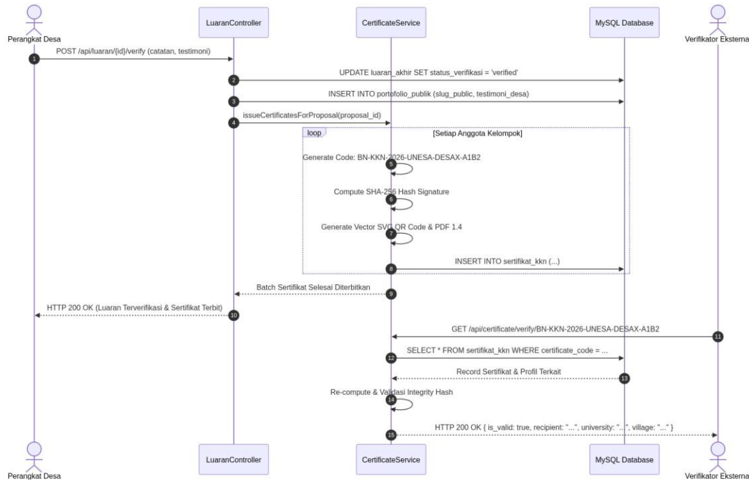
Gambar 5.7: Sequence Diagram Pengesahan Luaran & Verifikasi Publik
