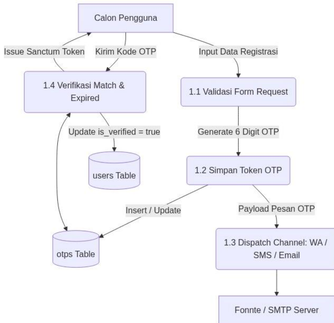
Gambar 3.3: DFD Level 2 - Proses 1.0 (Autentikasi & Verifikasi OTP)
