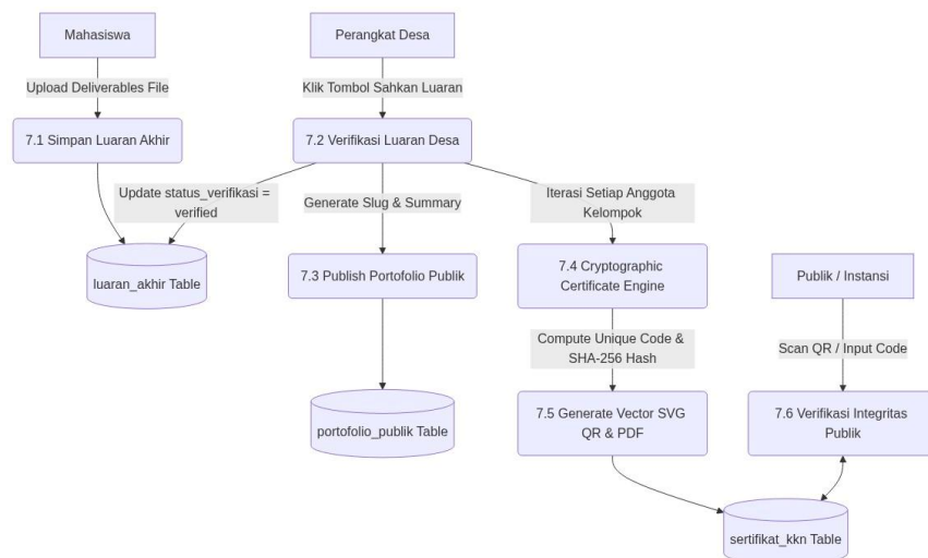
Gambar 3.5: DFD Level 2 - Proses 7.0 (Pengesahan Luaran & E-Sertifikat)
