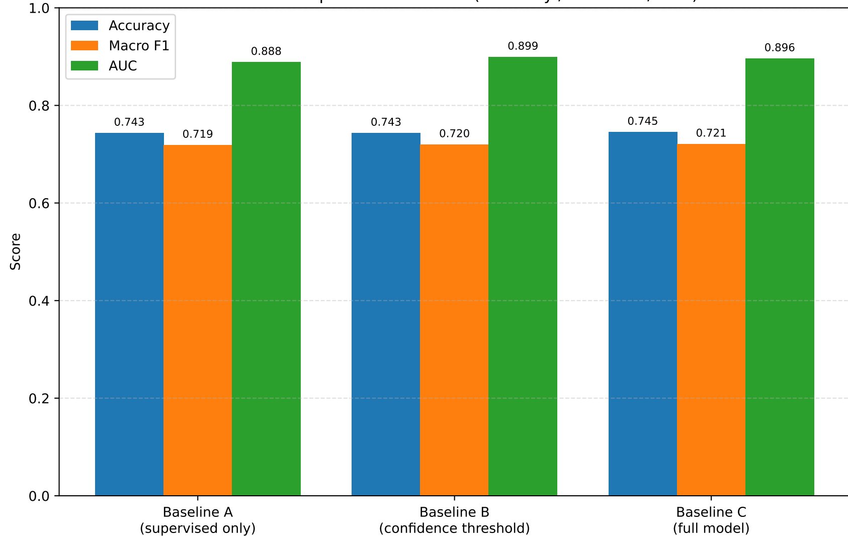
Ablation Comparison — Test Set (Accuracy / Macro F1 / AUC)
