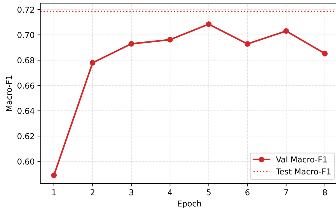
Macro-F1
