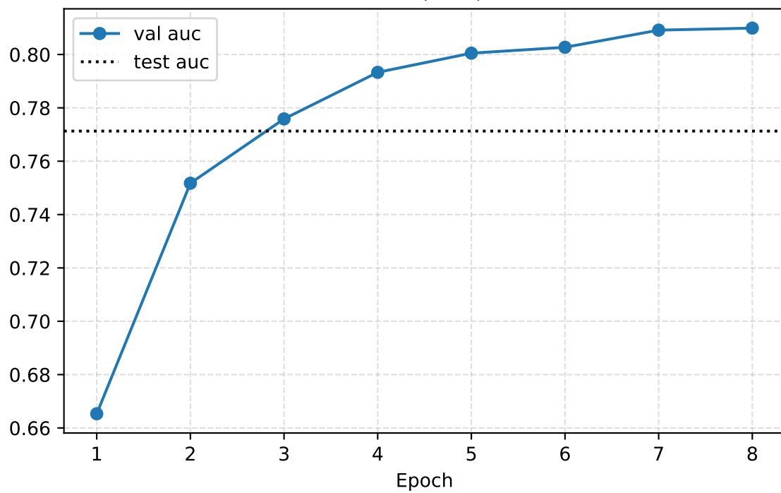
AUC (OvR)
