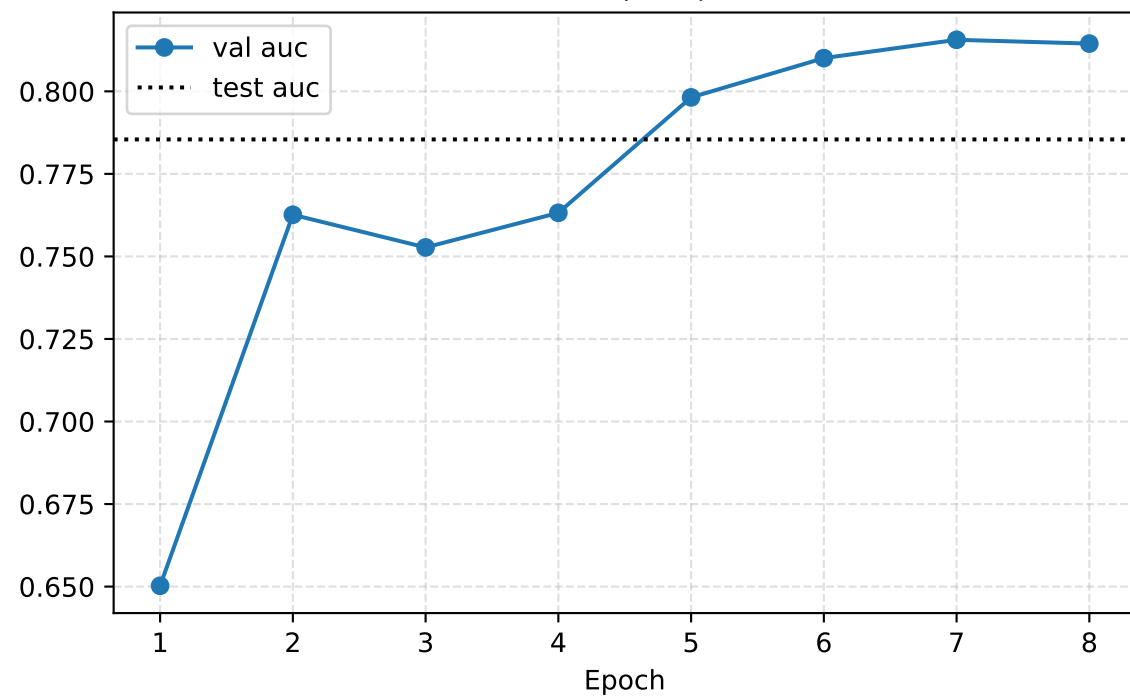
AUC (OvR)
