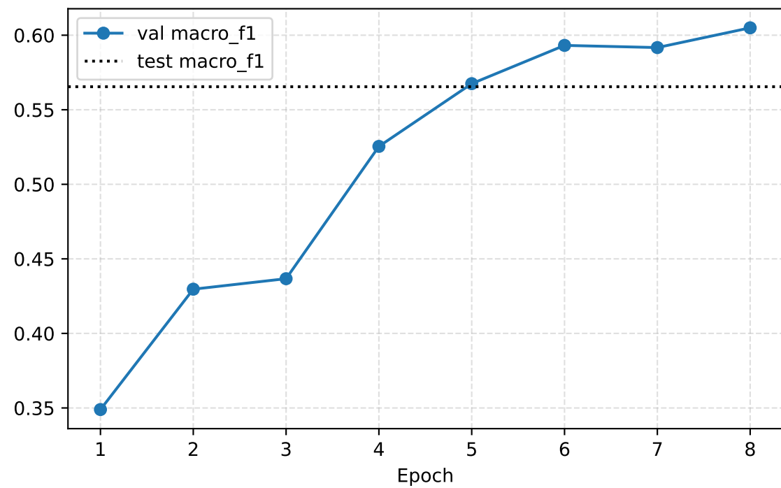
Macro-F1
