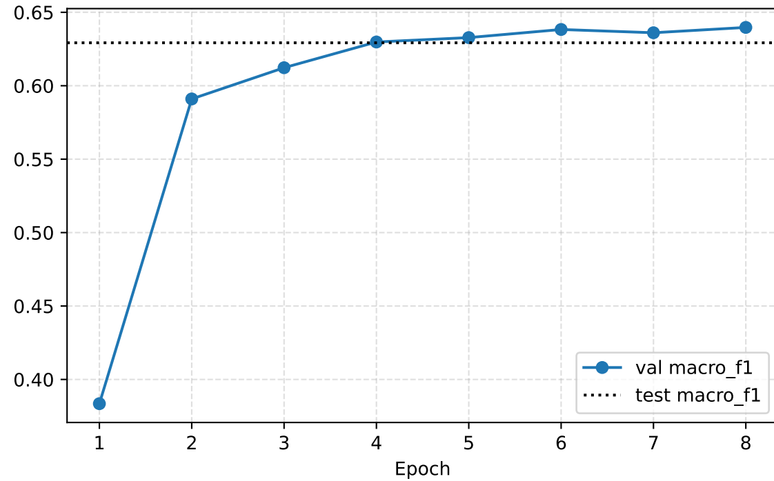
Macro-F1
