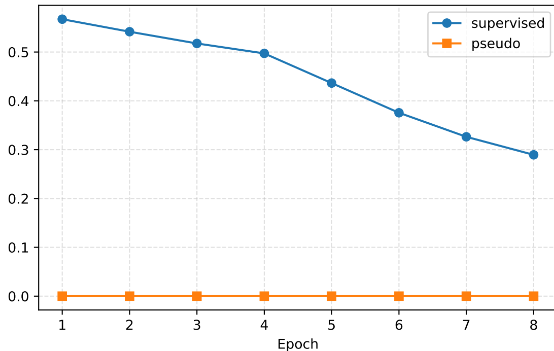
Macro-F1
