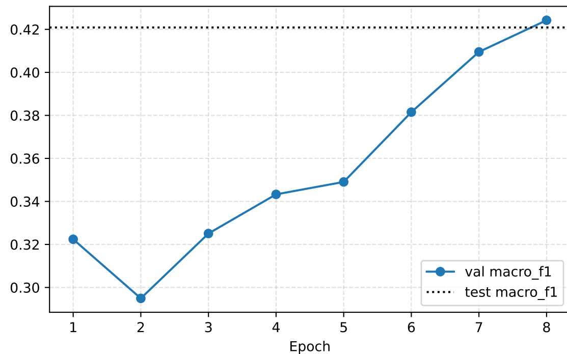
Macro-F1
