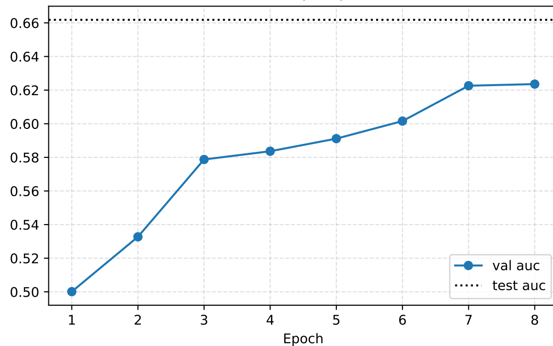
AUC (OvR)
