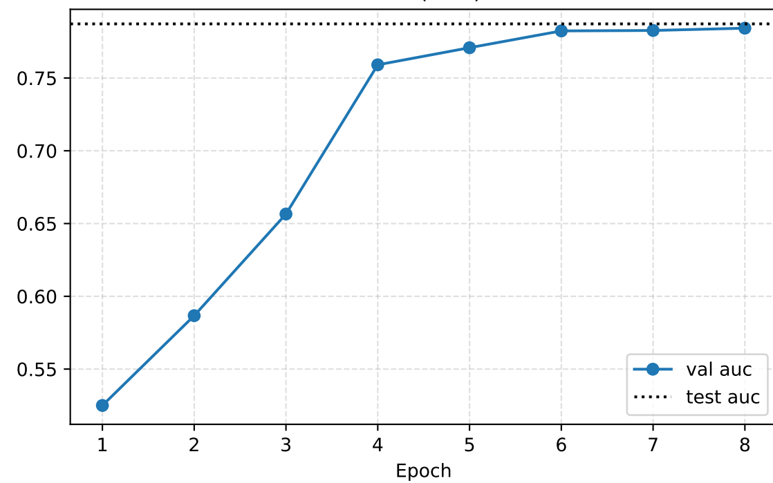
AUC (OvR)
