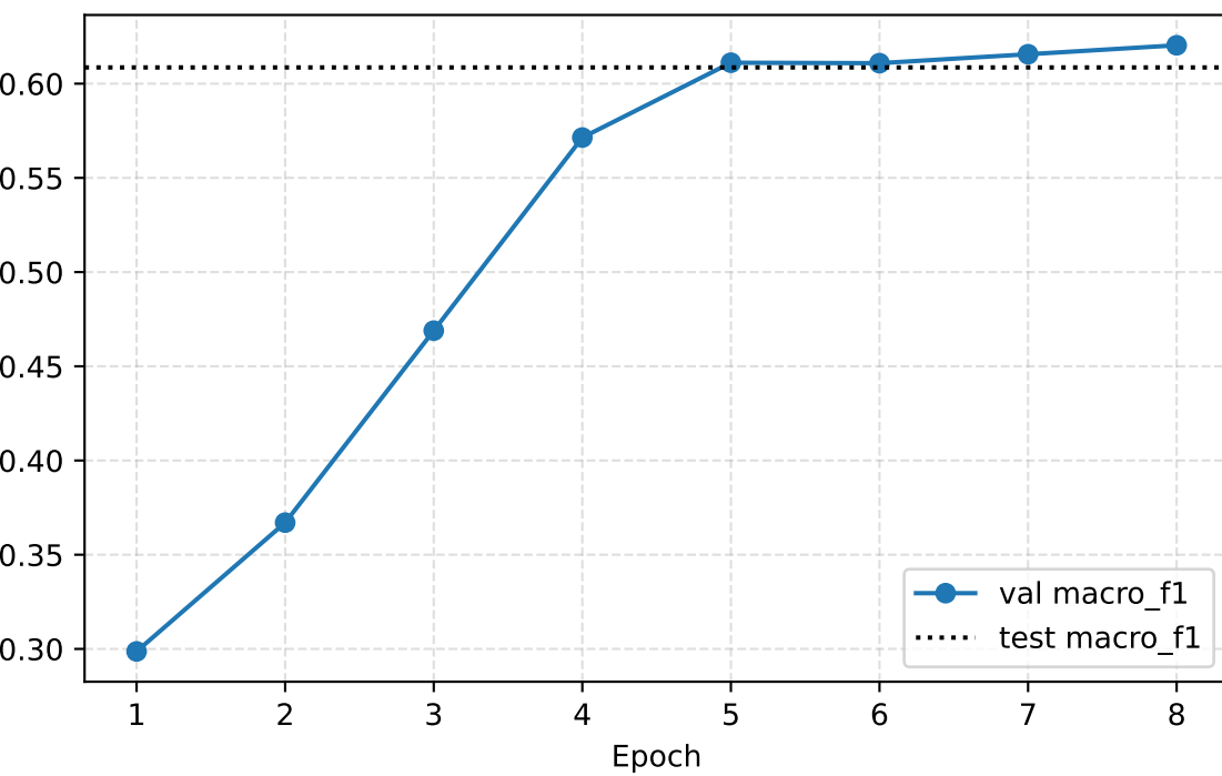
Macro-F1
