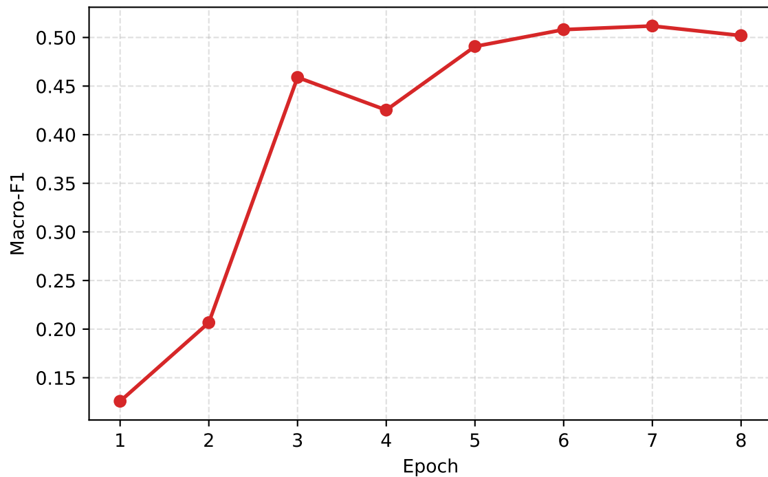
Validation Macro-F1
