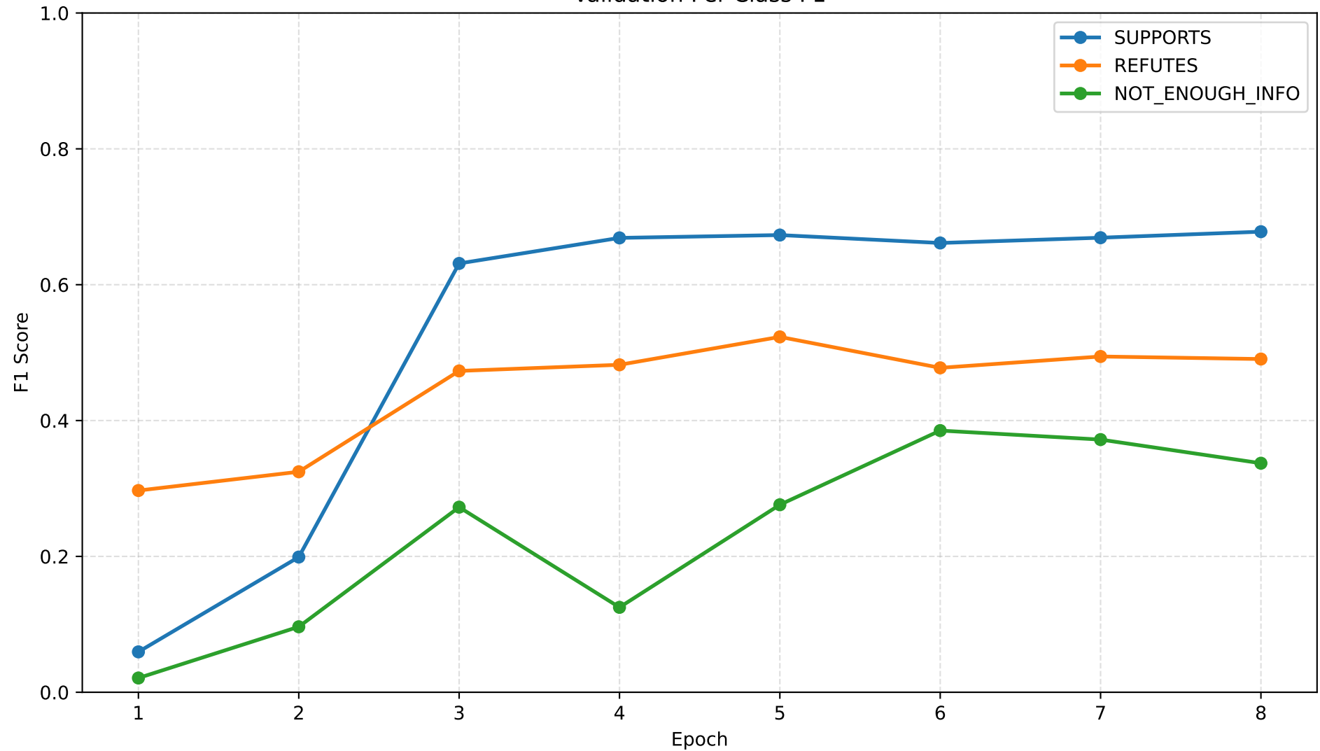
Validation Per-Class F1
