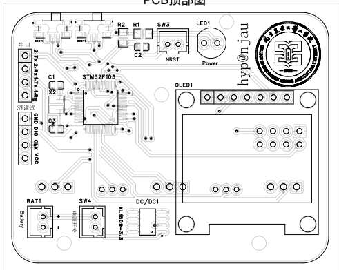
PCB顶部图
