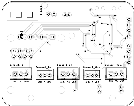
PCB底部图
