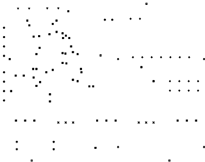
PCB打孔图
