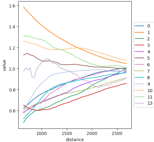
\frac{p(exp|1)}{p(exp)}
