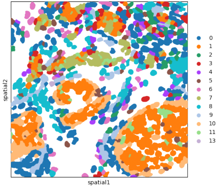
leiden
